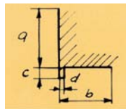
607 Rechtwinkel- und Schlitzschnitt a = 100 mm b = 115 mm c = 0-20 mm d = 2 mm
