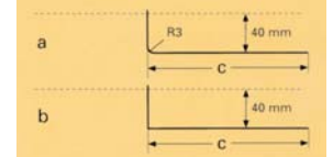
633 Rechtwinkelausschnitt c = 200 / 300 / 400 mm
