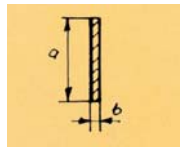
608 Schlitzschnitt a = max. 115 mm b = 2 mm
