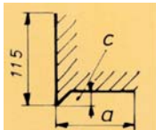
605 Rechtwinkelschnitt mit Hefrand a = 115 mm c = 15 mm
