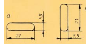
627 Bandschlitz abgerundet
