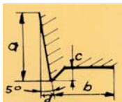
606 Stumpfwinkel- schnitt mit Hefrand a = 115 mm c = 15 mm b = 115 mm d = 10 mm
