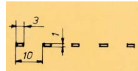
629 Mehrfach Schlitzlochung
