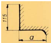
604 Rechtwinkelschnitt auf Rundung a = 30 - 100 mm
