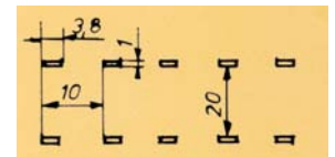
630 Doppelte Mehrfach-Schlitz- lochung 32 Paar Schlitz 3,8 x 1 mm
