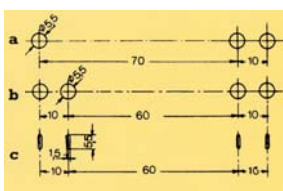
303 Mehrfachlochung
