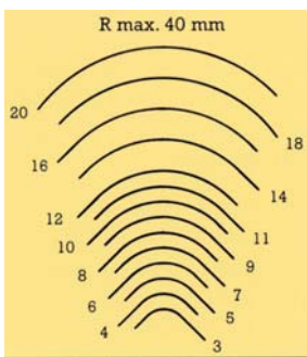
301 Eckenrundung
