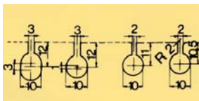
304 / 305 / 306 / 306a Registerkartenschnitte
