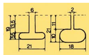
315 / 316 Registerkartenschnitte
