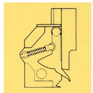
318 Eckeneinziehwerkzeug mit Kralle, Radius nach Wahl
